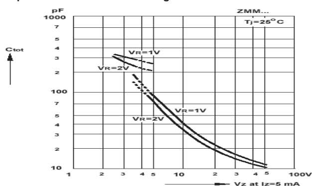
Capacitance versus Zener voltage
